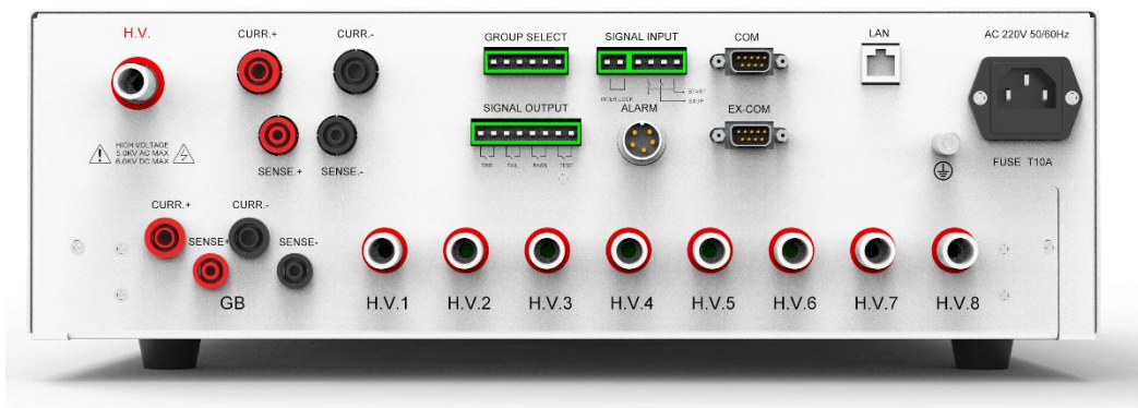
HEX305 后面板
